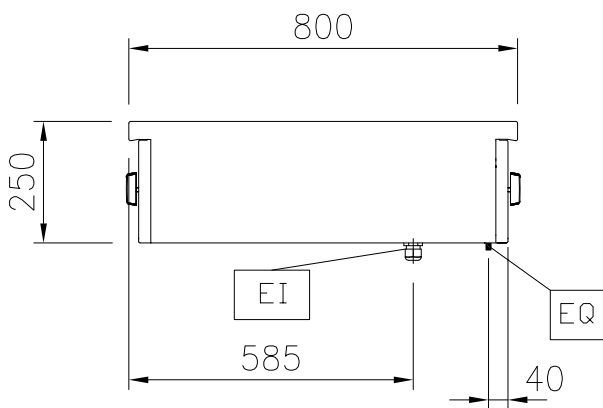
Zij aanzicht
