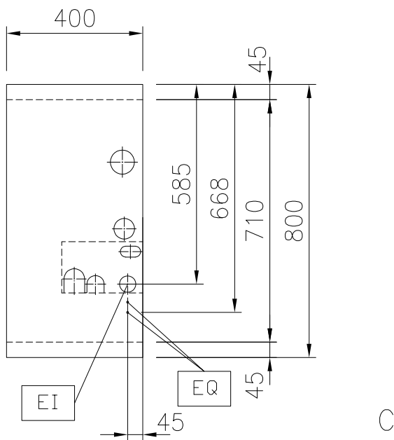
Boven aanzicht
